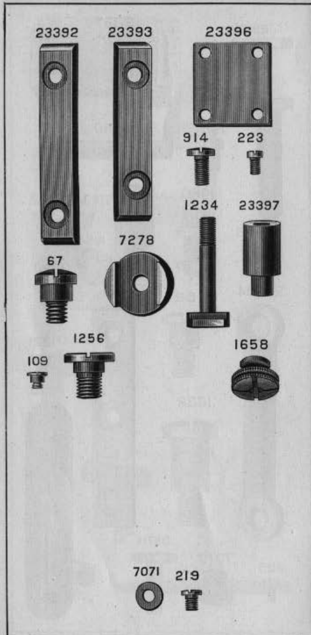
PLATE 4008—FULL SIZE
