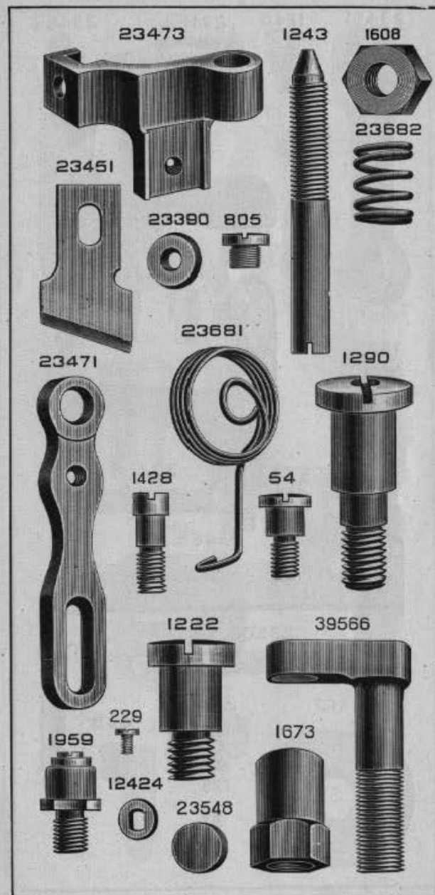
PLATE 4014—FULL SIZE
