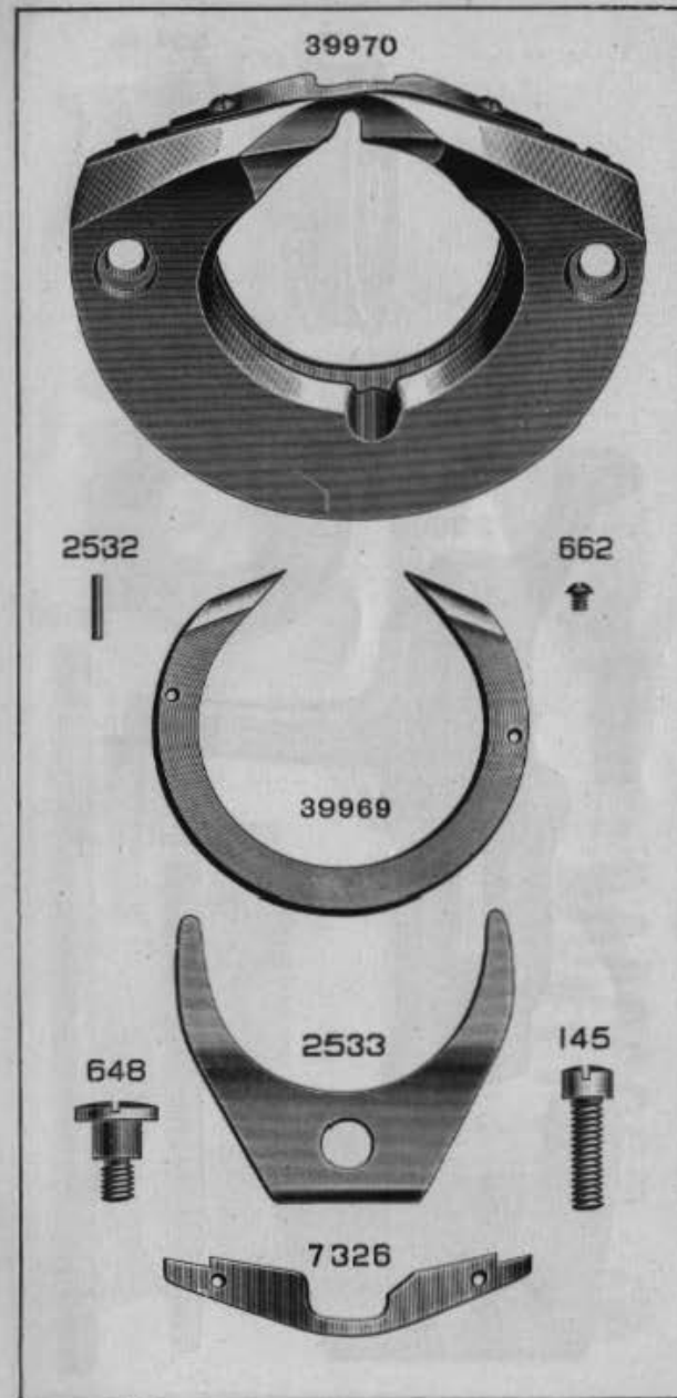
PLATE 4018—FULL SIZE
