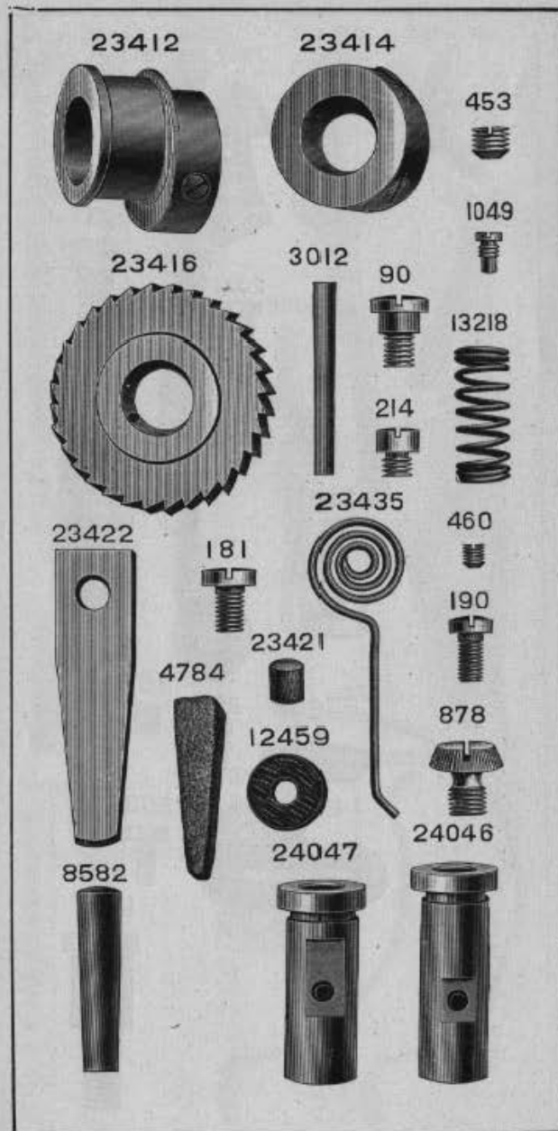
PLATE 4013—FULL SIZE
