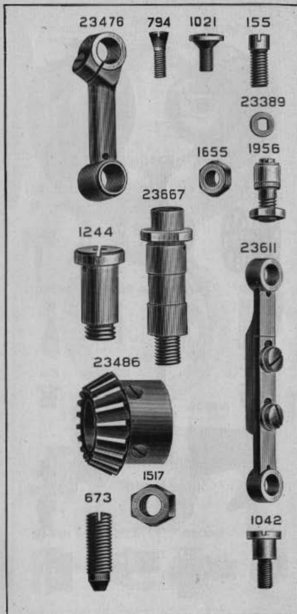
PLATE 4016—FULL SIZE
